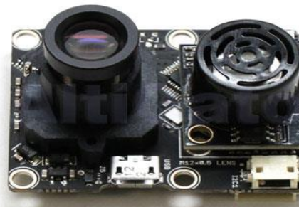
(d) Optical Flow sensor
